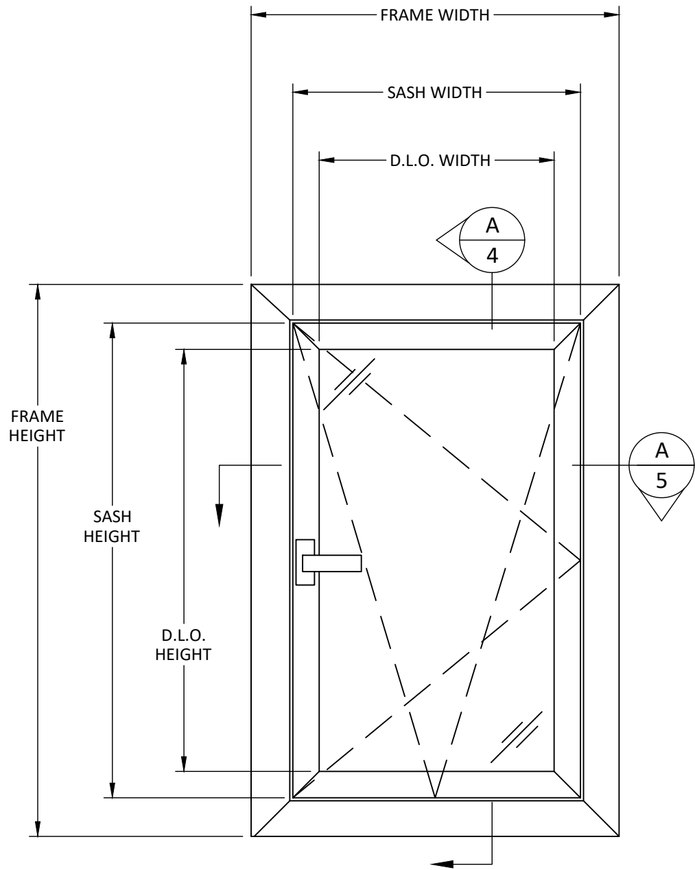
ELEVATION
